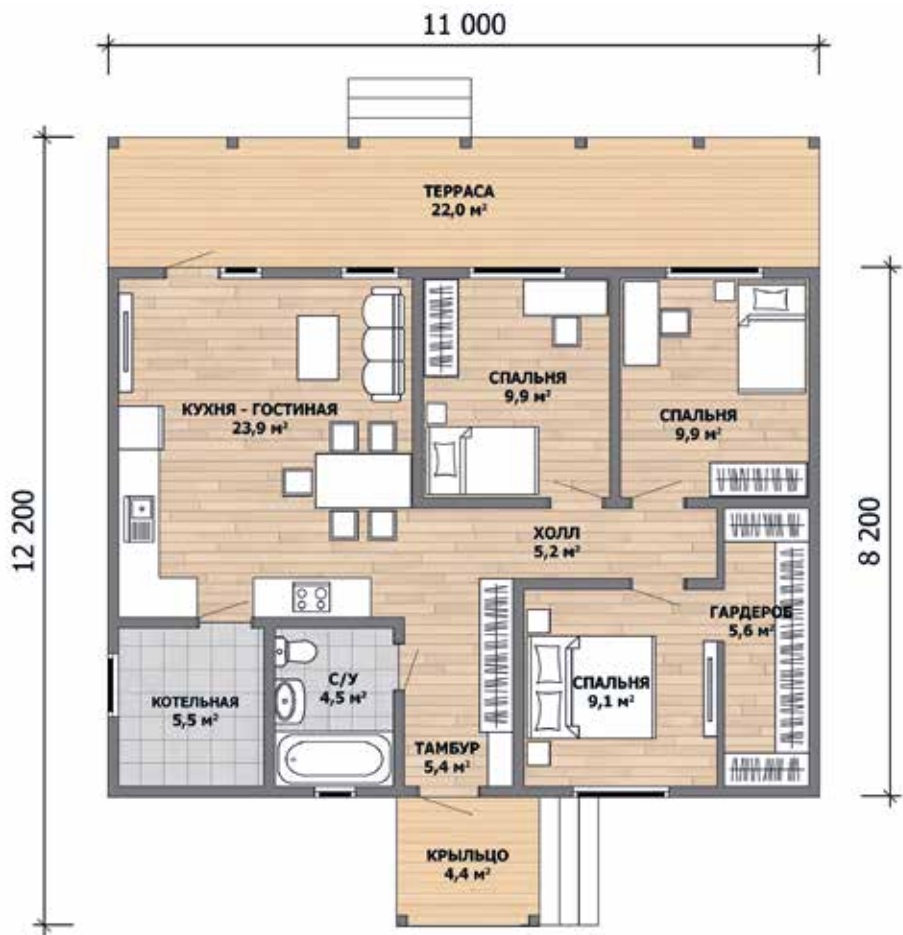
ПЛАН ЭТАЖА
